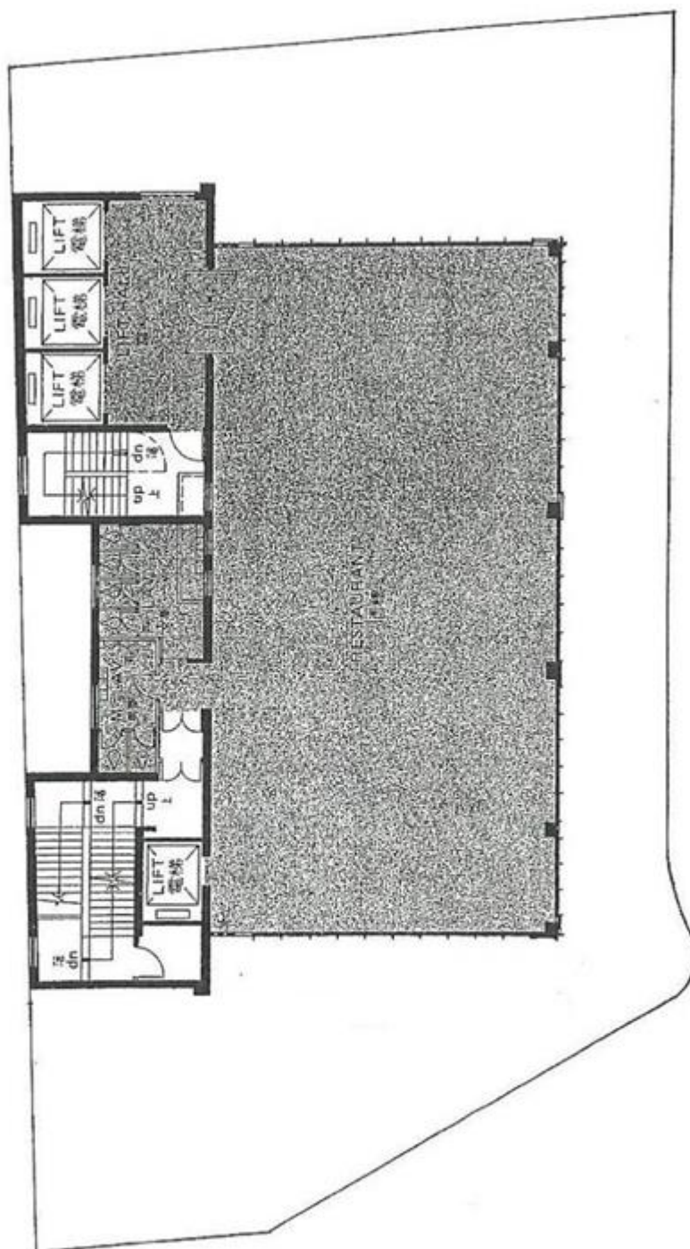
15TH FLOOR PLAN 十五樓平面圖
